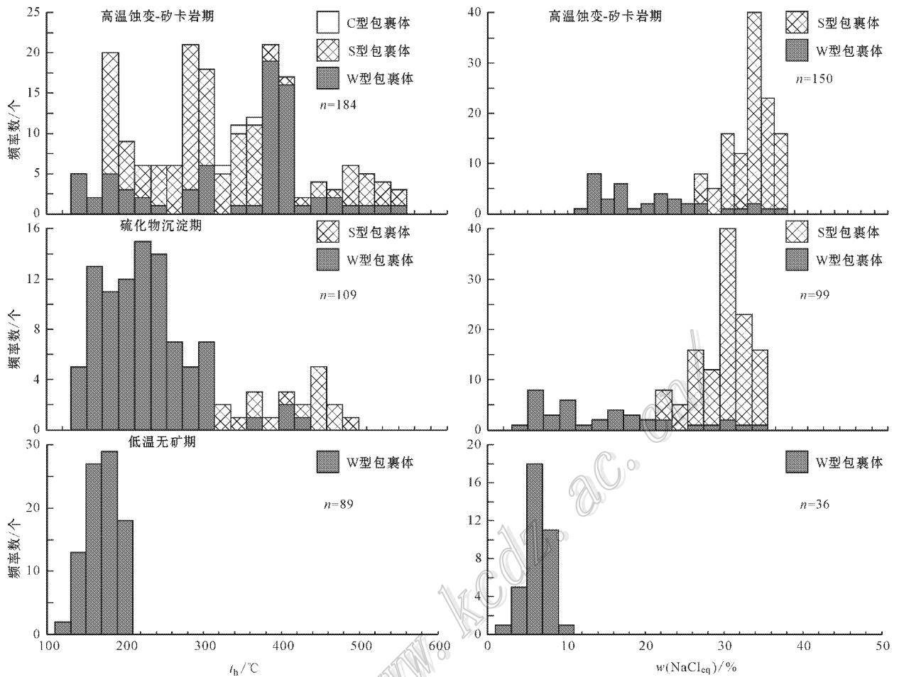
图6 秋树湾铜钼矿流体包裹体均一温度及盐度直方图
