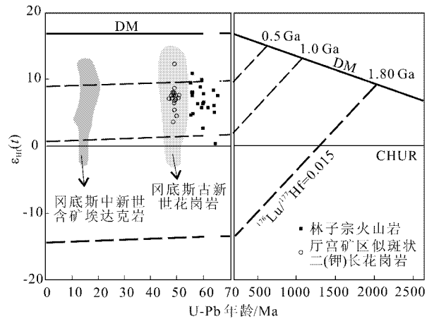
图 7 厅宫矿区始新世斑状二长花岗岩锆石 \epsilon_{\text{Hf}}(t) (U-Pb) 年龄图解 (底图据 Chu et al., 2006 修改; 林子宗火山岩据李皓扬 (2007); 冈底斯古新世—始新世花岗岩据 Ji 等 (2009); 冈底斯中新世埃达克岩据 Chung 等 (2009); Xu 等 (2010); 杨志明 (2008b); Yang 等 (2009))
