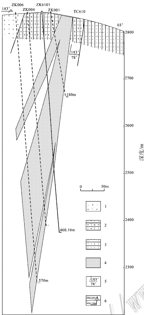
图 11 松湖矿区 0—0' 勘探线剖面图(据①修改)
