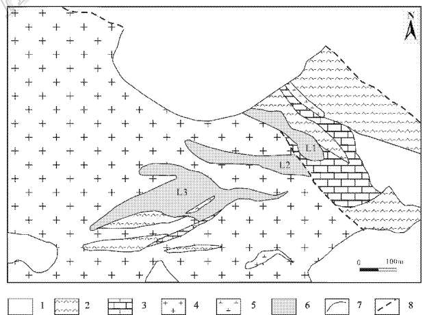
图2 备战铁矿区地质图(据①修改)
