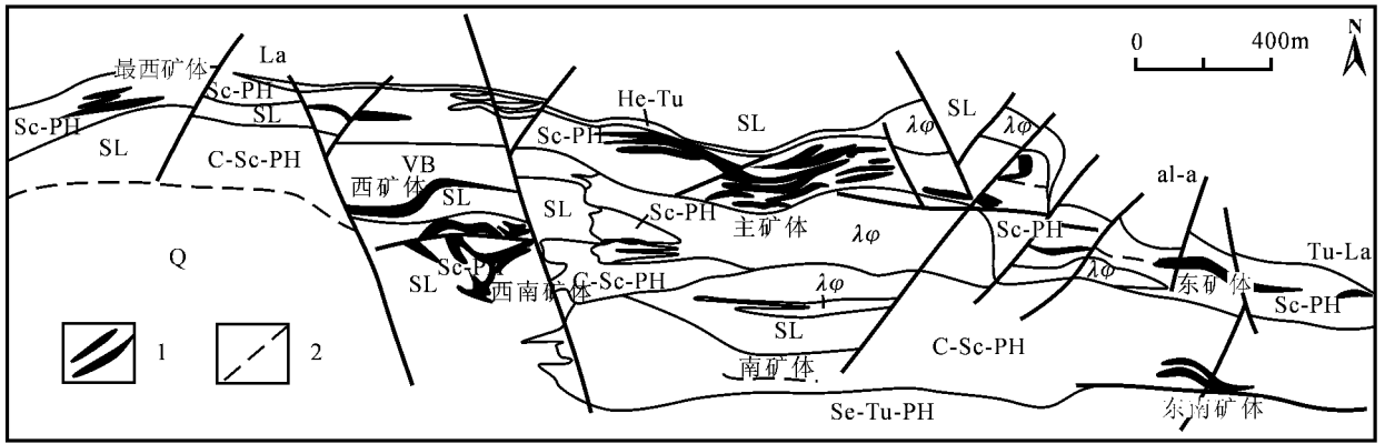
图 12 式可布台矿区地质图(据田培仕,1990 修改)
