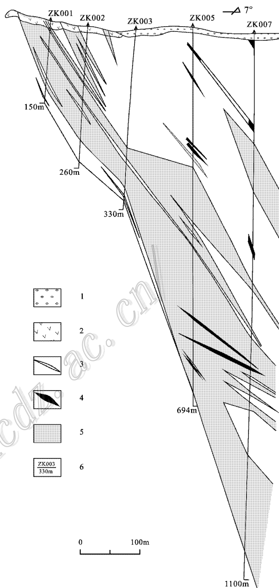
图 3 备战铁矿 0—0' 勘探线剖面图
