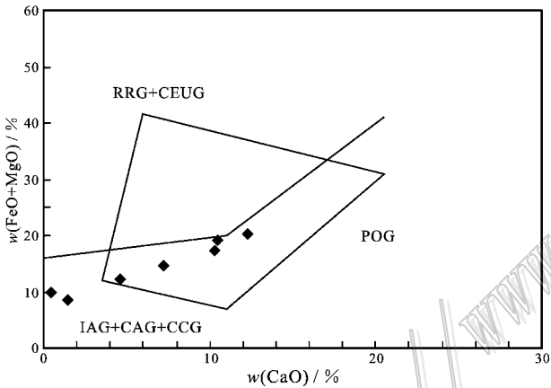
图 6 千家岩体花岗岩构造判别图 (Maniar et al., 1989) POG—后造山花岗岩; RRG—裂谷花岗岩; CEUG—大陆造陆抬升花岗岩; CAG—大陆弧花岗岩; CCG—大陆碰撞花岗岩; IAG—岛弧花岗岩
