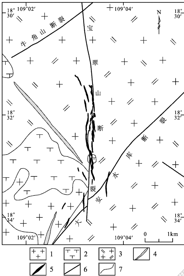
图 2 后万岭铅锌矿矿区地质简图
