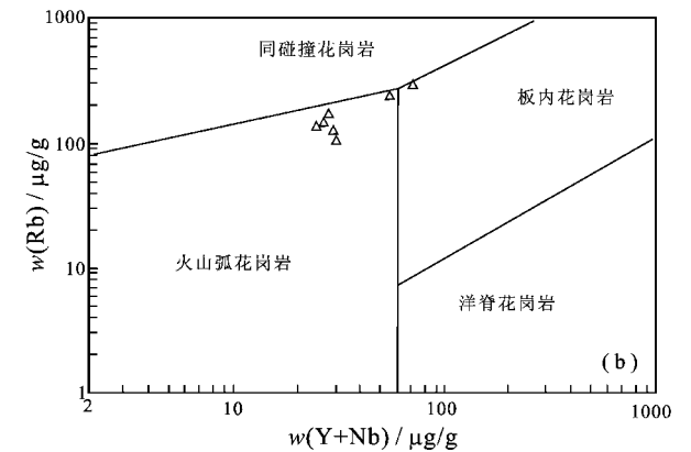
图 7 千家岩体花岗岩源区及构造判别图 (据 Pearce, 1996 修改)
