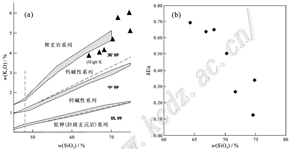
图 3 千家岩体花岗岩类 \text{SiO}_2\text{-K}_2\text{O} 图解 (a) (Morrison, 1980) 和 \delta\text{Eu-SiO}_2 图解 (b)
