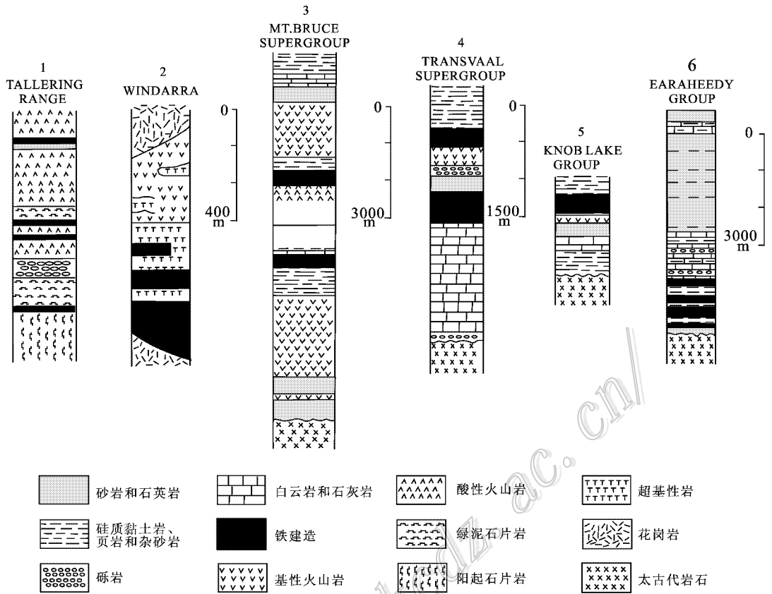
图 5 典型铁建造综合剖面图( 改自 Klein 2005 )
