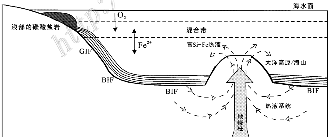
图 4 BIF 和 GIF 沉积环境示意图( 改自 Wang et al., 2009 和 Bekker et al., 2010) 地幔柱成因的科马提岩与海底热液相互作用析出 Si 和 Fe, 交替沉淀形成了铁建造
