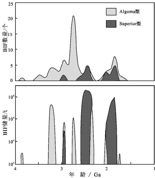
图2 两类BIF在不同时间的变化趋势图 (改自Huston et al., 2004)
