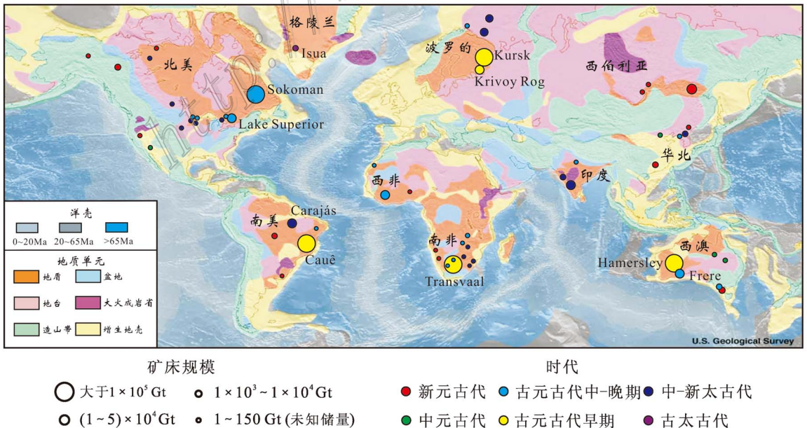
图3 全球主要IF及古老克拉通分布图(改自Trendall, 2002和Bekker et al., 2010)
