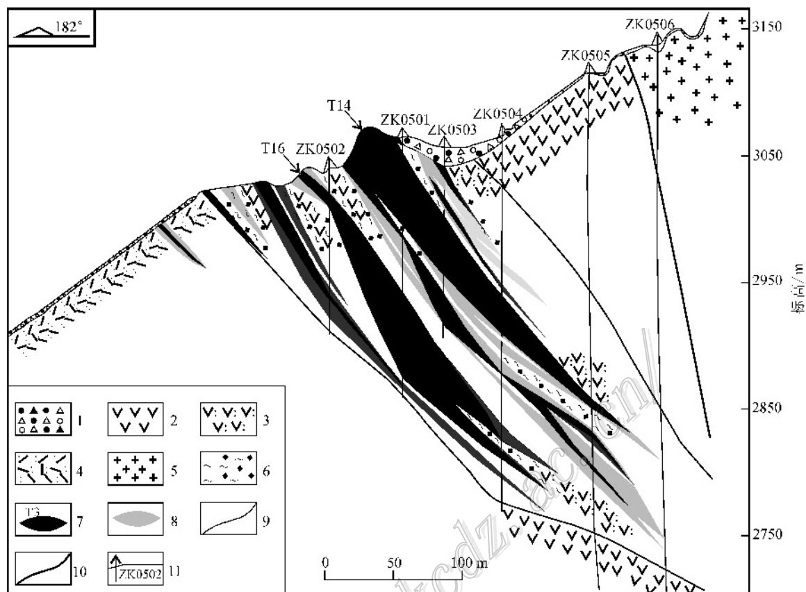
图3 阿克萨依铁矿区东矿段第5勘探线剖面图(据四川省地质矿产勘查开发局四〇五地质队,2011 修改)
