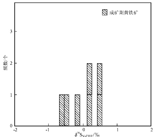
图9 阿克萨依铁矿床黄铁矿硫同位素直方图
