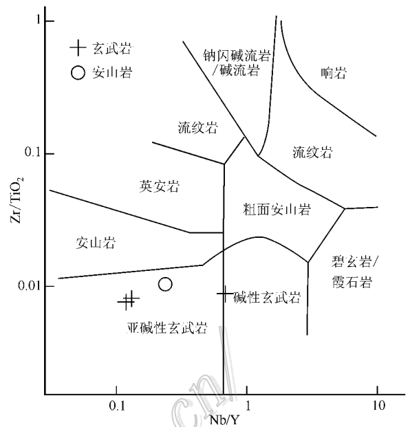
图6 阿克萨依铁矿区火山岩Nb/Y-Zr/TiO 2 图解 (据Floyd et al., 1978)
