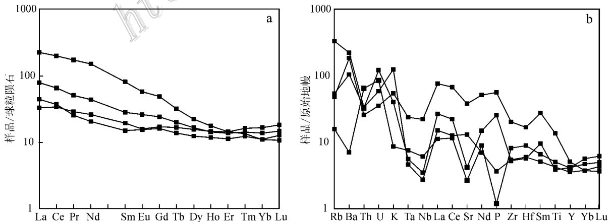
图 7 阿克苏依铁矿区火山岩稀土元素球粒陨石标准化配分图 (a) 和微量元素原始地幔标准化蛛网图 (b) (标准化值据 Sun et al., 1989)
