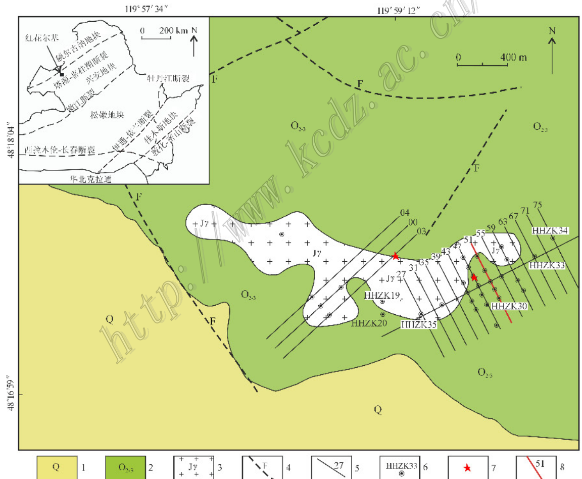
图1 红花尔基钨多金属矿床区域位置图及矿区地质图
