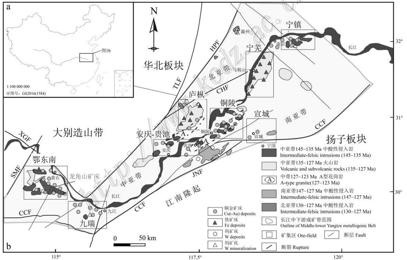
图 1 长中下游成矿带矿床分布示意图(据常印佛等, 1991;周涛发等, 2017)
