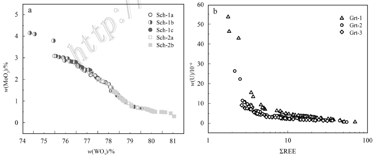
图 9 龙角山矿床白钨矿和石榴子石主、微量元素图解
