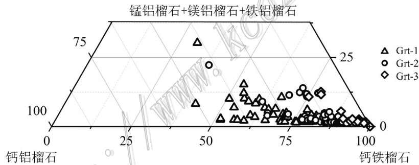
图8 龙角山矿床石榴子石三角图
