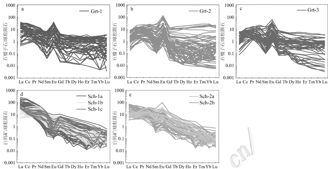
图10 龙角山矿床白钨矿和石榴子石稀土元素配分图解
