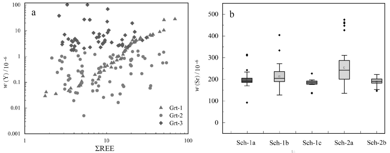
图11 龙角山矿床石榴子石和白钨矿图解
