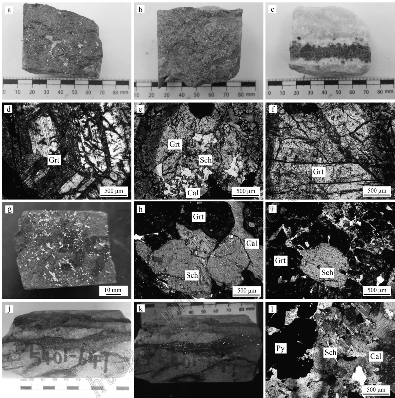
图6 龙角山矿床手标本和镜下照片
