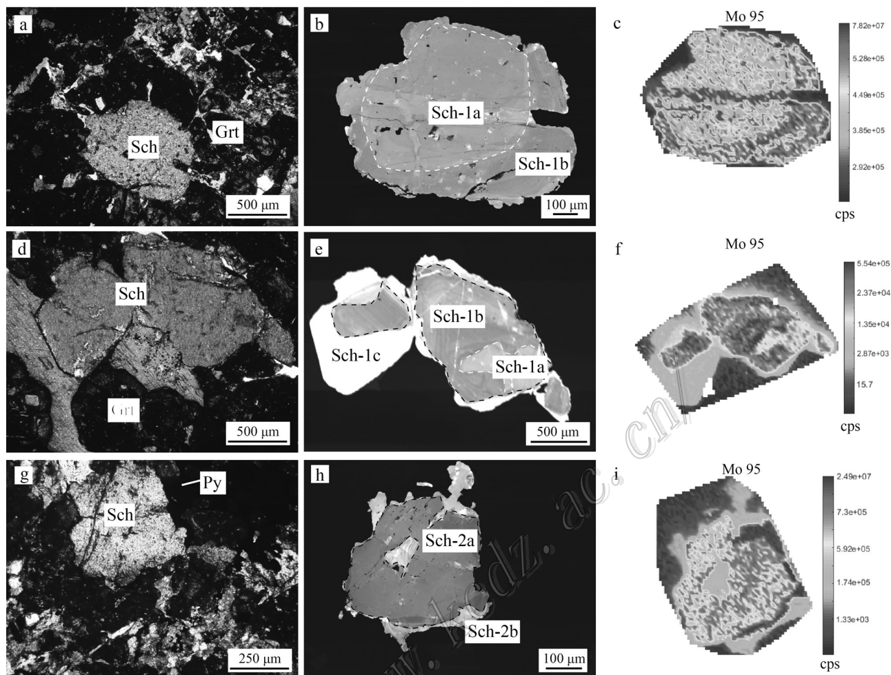
图7 龙角山矿床白钨矿阴极发光和面扫描特征
