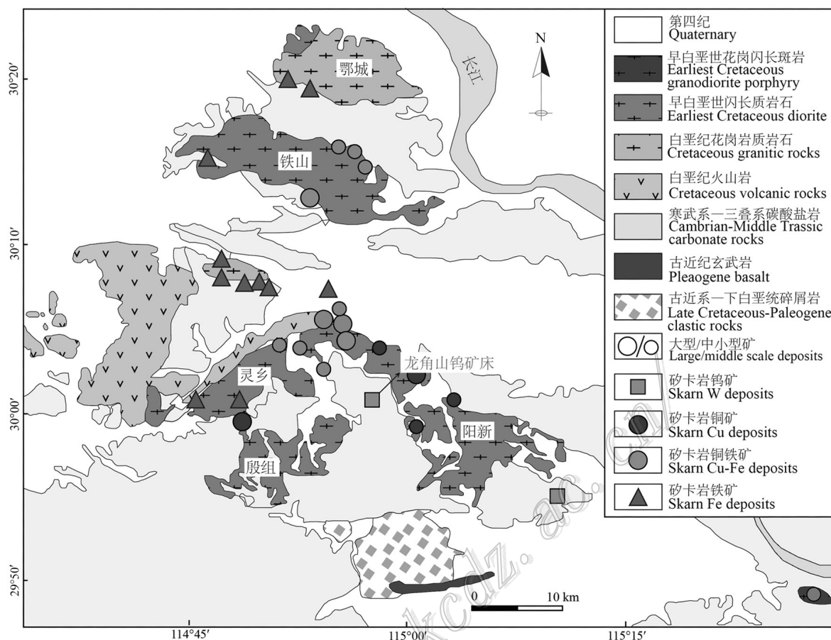
图2 鄂东南矿集区地质简图(据谢桂青等,2008修改)
