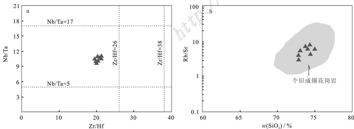
图 7 Nb/Ta-Zr/Hf 判别图解 (a, 根据吴福元等, 2017 修改) 和 Rb/Sr- w(SiO_2) 判别图解 (b, 根据解世熊, 2021 修改)
