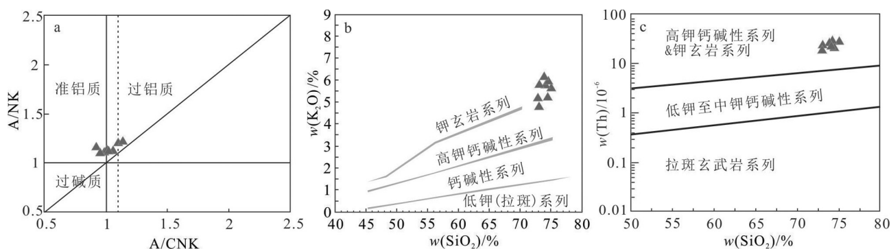
图 6 A/NK-A/CNK 判别图解 (a, 底图据 Frost et al., 2001)、 w(K_2O)-w(SiO_2) 图解 (b, 底图据 Peccerillo et al., 1976) 和 w(Th)-w(SiO_2) 图解 (c, 底图据 Hastie et al., 2007)
